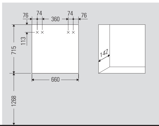
Kivágás mérete beépített szekrények számára
